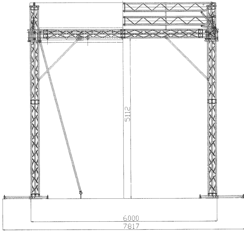
Rysunek 2. Widok zadaszienia z boku
